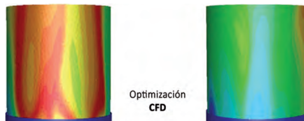
FIGURA 5. Distribución de temperaturas antes y después de la optimización
